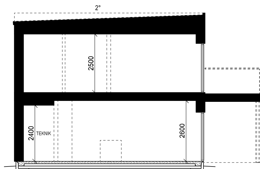
SEKTION B-B
