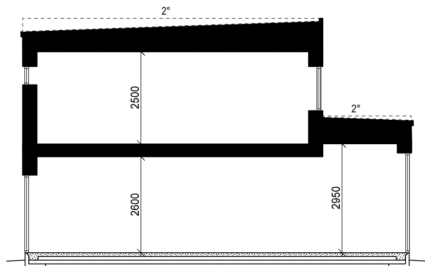
SEKTION A-A
