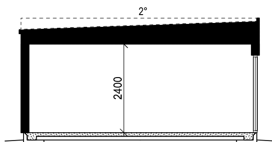
SEKTION A-A
