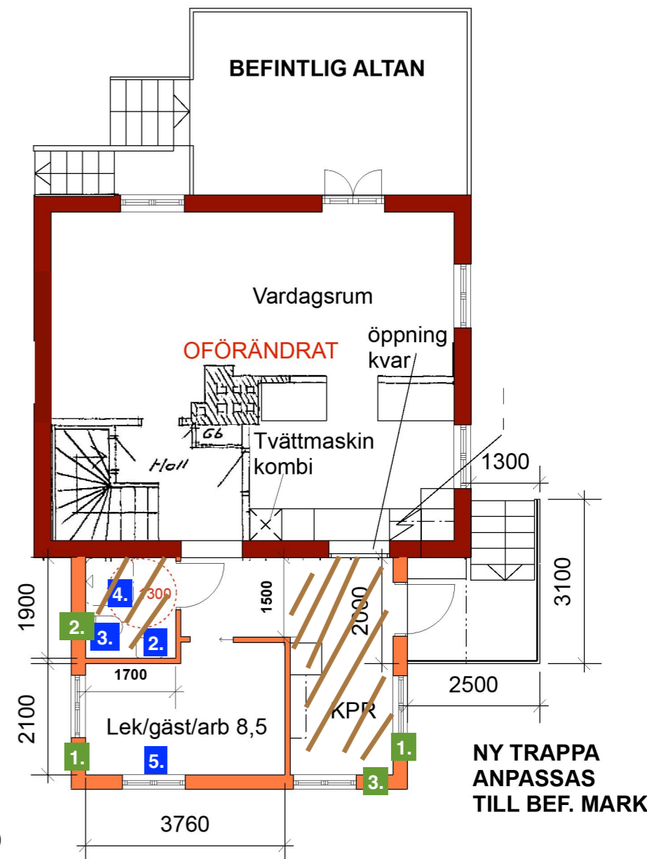
ENTRÉPLAN BV
