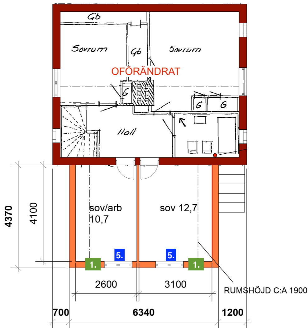
ÖVRE PLAN 1 TR
