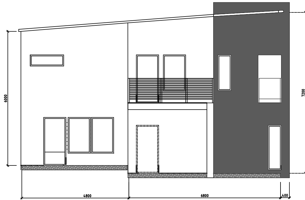
Fasad Väst
