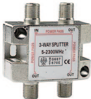
Clas Ohlson Art nr: 22-3689 3-vägs. Dämpning 7 dB 5-2300 Mhz
