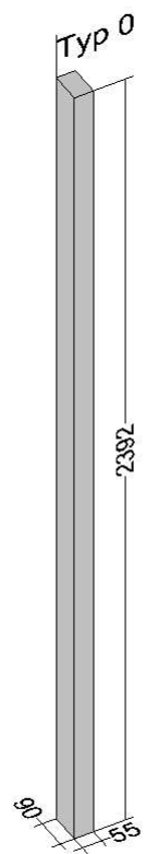
Det E - LIMTRÄSTOLPE 55X90X2500 MM
