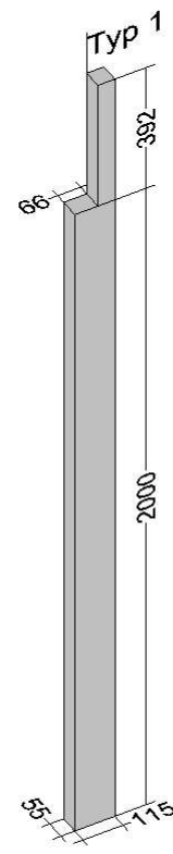
Det H - LIMTRÄSTOLPE 55X115X2500 MM
