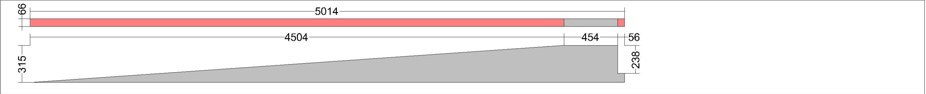
Det 7RA - LIMTRÄBALK 66X315X6200 MM
