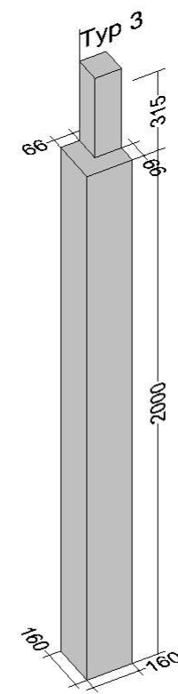
Det K - LIMTRÄSTOLPE 160X160X2500 MM
