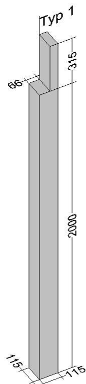
Det O - LIMTRÄSTOLPE 115X115X2500 MM
