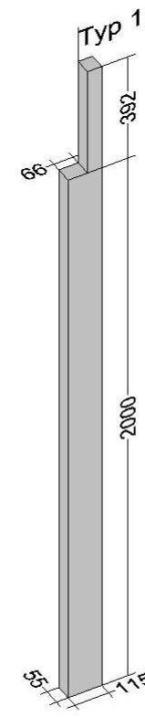
Det I - LIMTRÄSTOLPE 55X115X2500 MM
