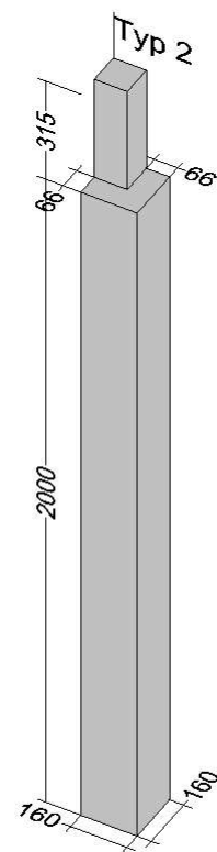
Det G - LIMTRÄSTOLPE 160X160X2500 MM
