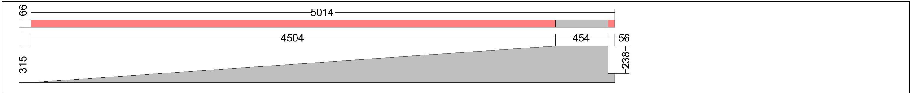
Det 7LA - LIMTRÄBALK 66X315X6200 MM
