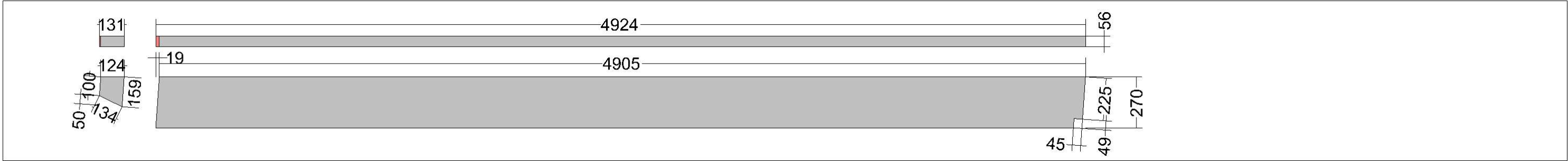
Det 6 - LIMTRÄBALK 56X270X6200 MM
