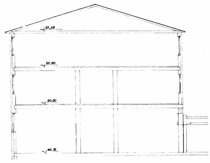
SEKTION GENOM LÅGDELEN
