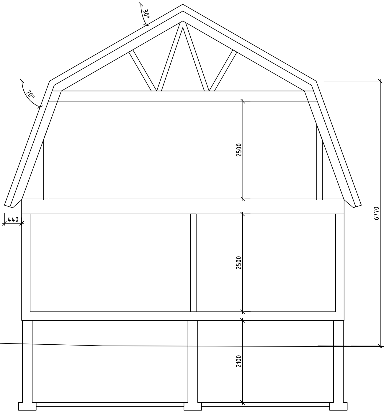
SEKTION A-A
