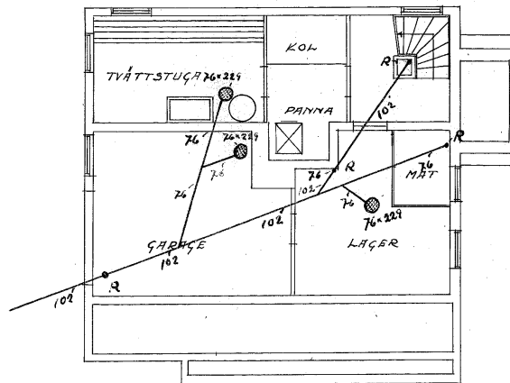
KÄLLARPLAN
