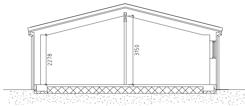
SEKTION B-B
