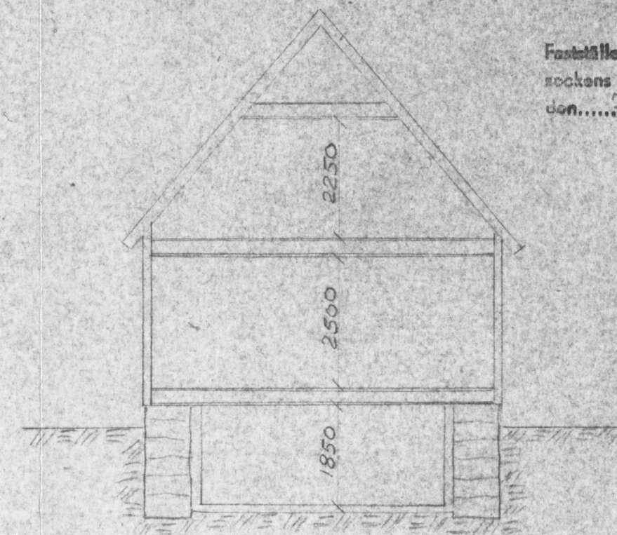
SEKTION
