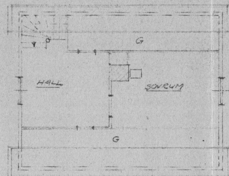
VINDSPLAN
