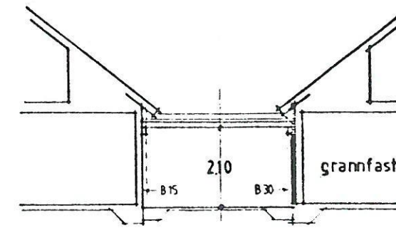
SEKTION GARAGE
