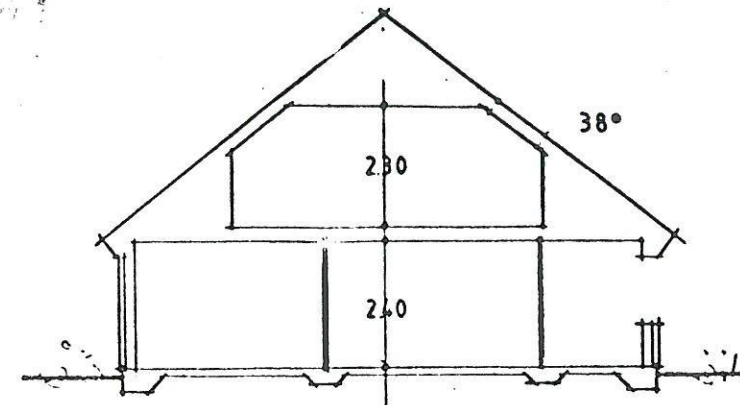
SEKTION
