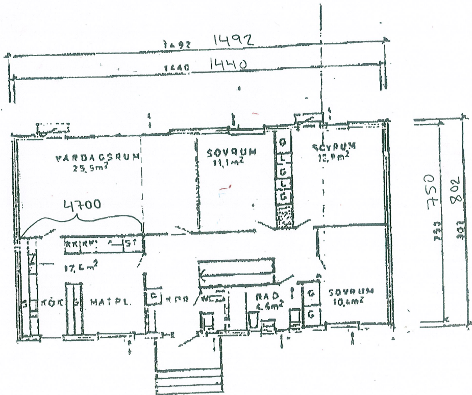
VÅNINGSPLAN 108,0m 2
