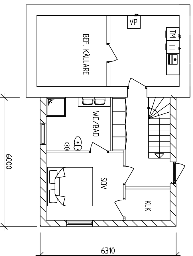
KÄLLARPLAN
