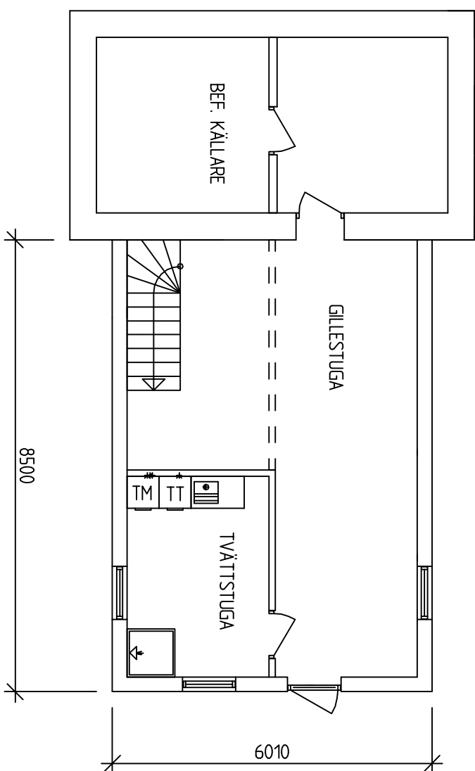
KÄLLARPLAN
