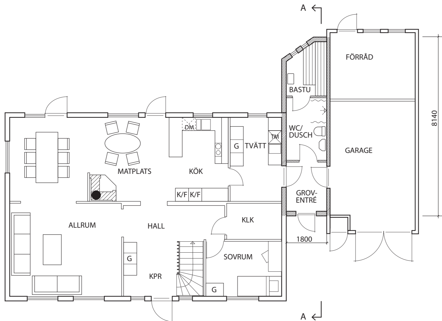
ENTRÉPLAN
