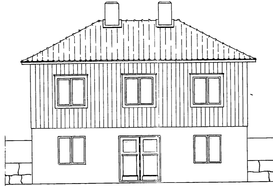
FASAD MOT VÄG
