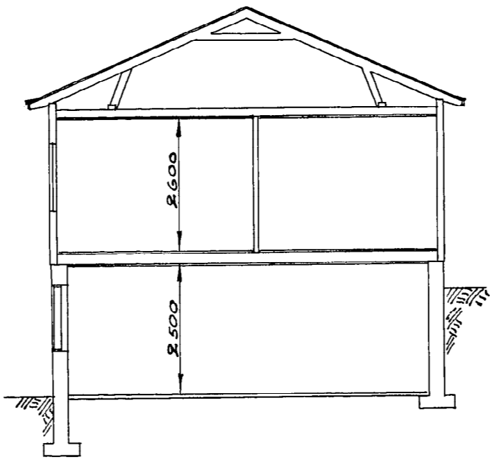
SEKTION A-B
