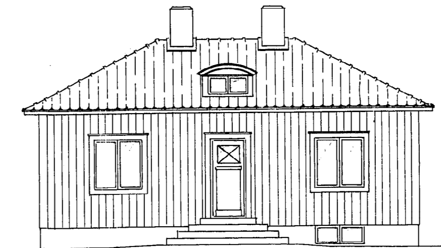
FASAD MOT GÄRD
