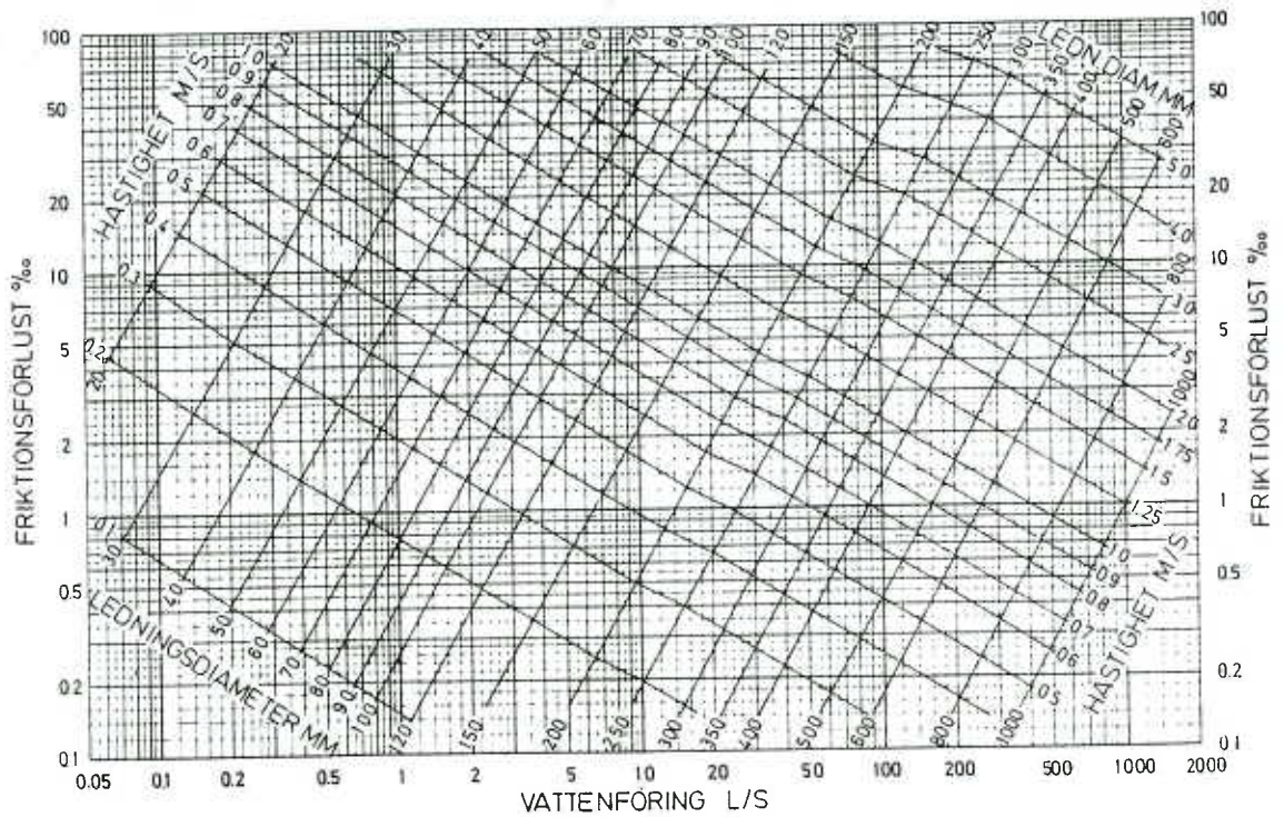
Figur 3.27 Friktionsförlustdiagram för vatten + 10°C. Rörtyp stål, Cu, Et, PE, PVC. k = 0,01 mm för diametern \leq 200 mm och k = 0,05 mm för diametern > 200 mm.
