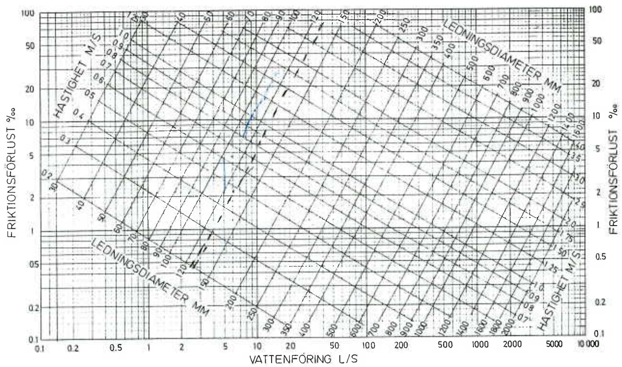
Figur 3.28 Friktionsförlustdiagram för vatten + 10°C. k = 0,1 mm. Rörtyp stål, gjut, AP
