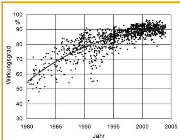
Abb. 3-1: Entwicklung der Kesselwirkungsgrade von hand- und automatisch beschickten Holzfeuerungen kleinerer Leistung seit 1980 – Ergebnisse aus Typenprüfungen bei Nenn- und Teilwärmeleistung (BLT Wieselburg)
