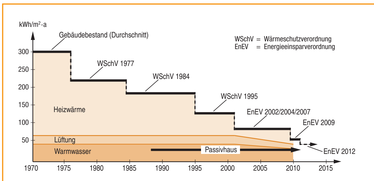
Abb. 2-1: Anforderungen an den Heizenergiebedarf in neugebauten Wohnhäusern
