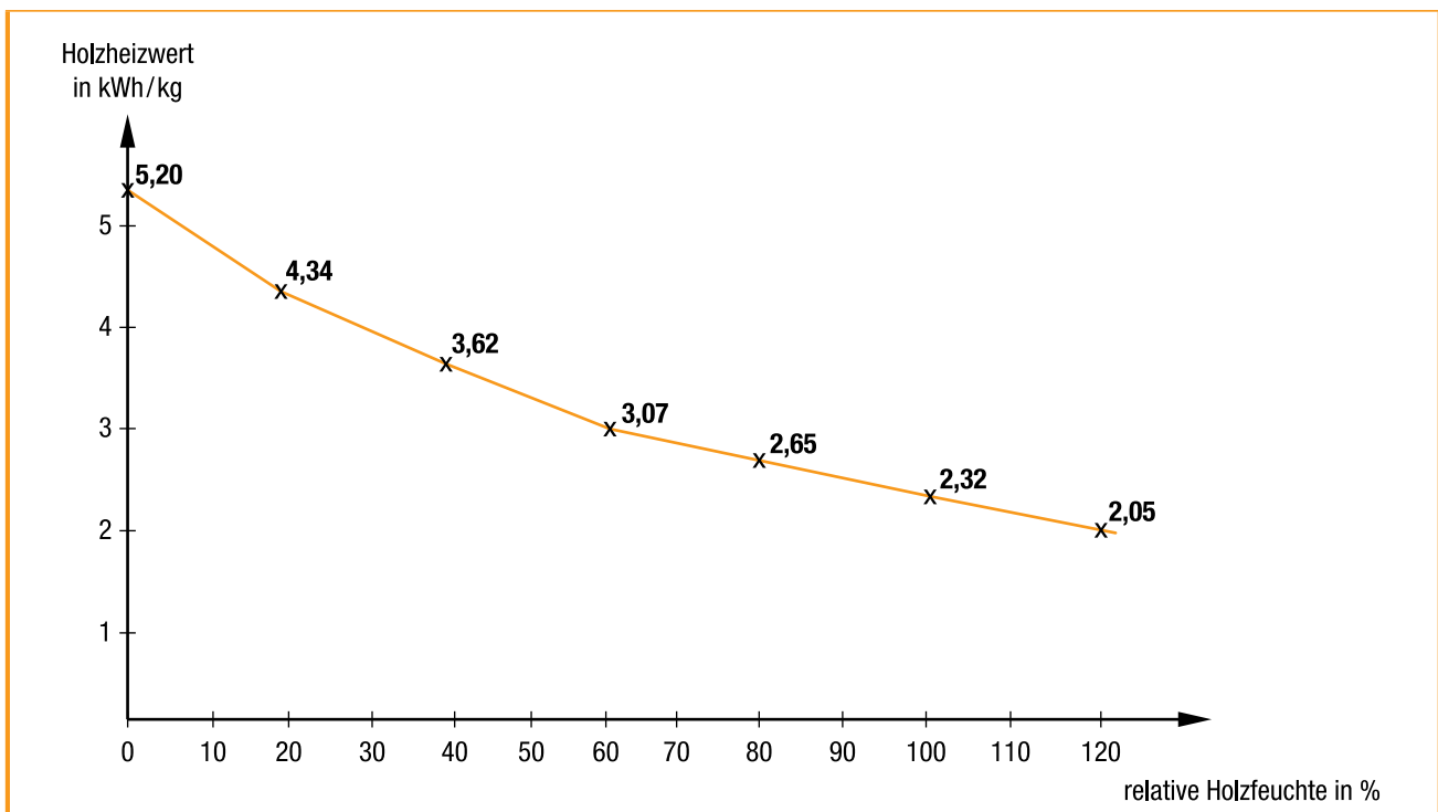
Abb. 2-3: Abhängigkeit des gewichtsbezogenen Holzheizwertes von der relativen Holzfeuchte
