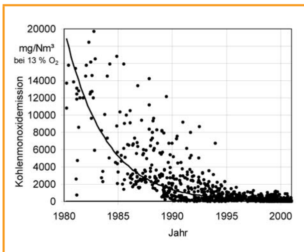
Abb. 3-2: Entwicklung der CO-Emissionen von hand- und automatisch beschickten Holzfeuerungen kleinerer Leistung seit 1980 – Ergebnisse aus Typenprüfungen bei Nenn- und Teilwärmeleistung (BLT Wieselburg)
