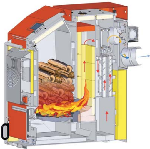
Fischer: Schnittmodell TX 33 bzw. TX 50
