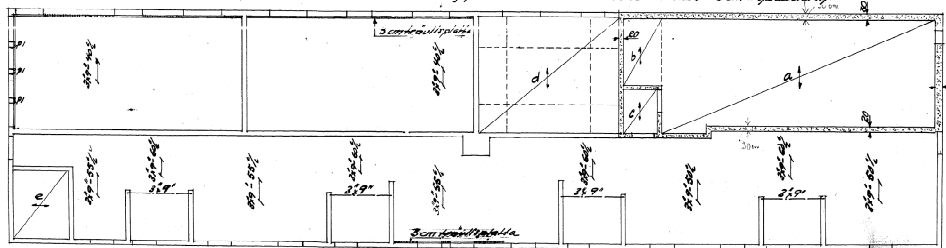
Bjälklag över källaren
