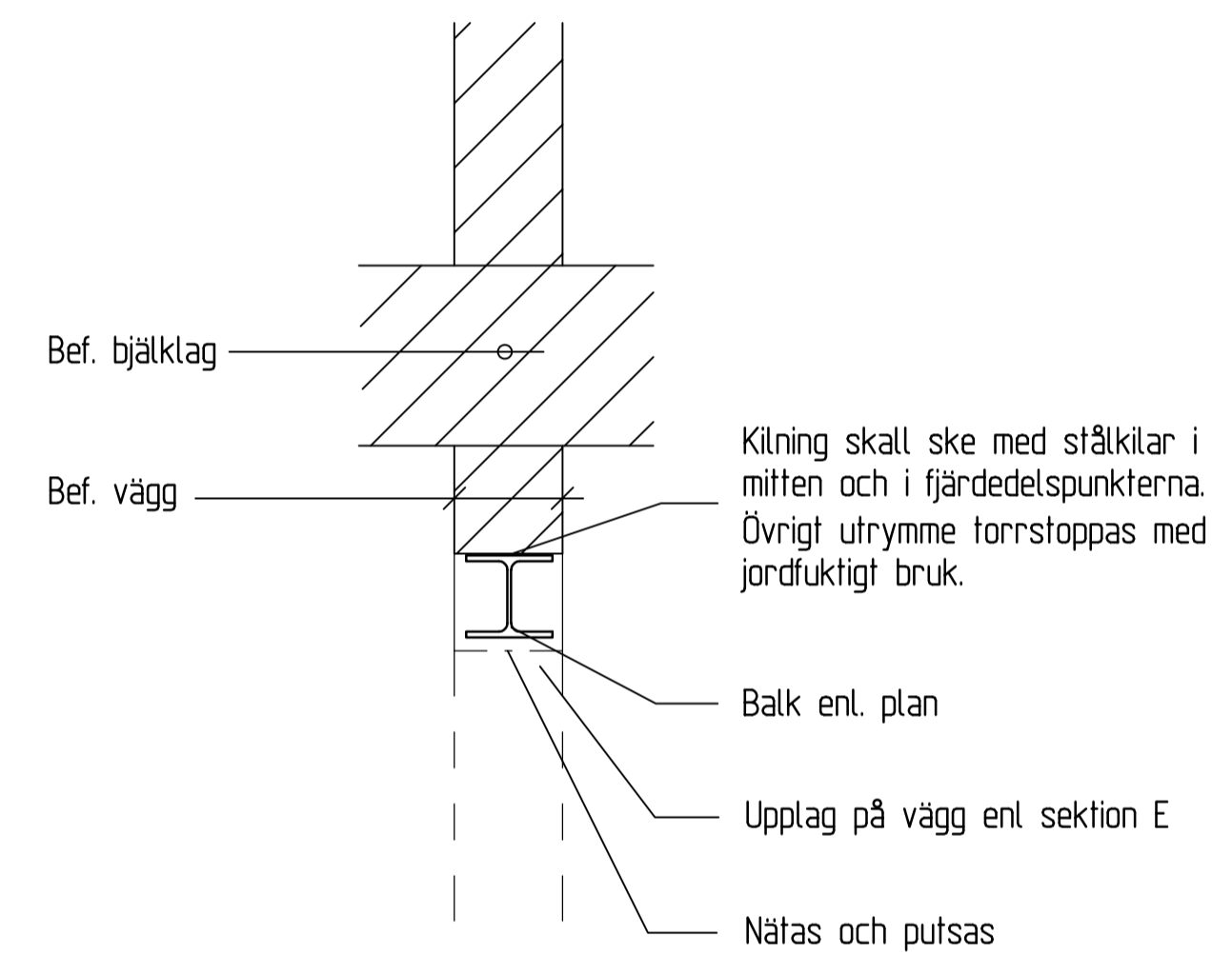
SEKTION B -1:10-
