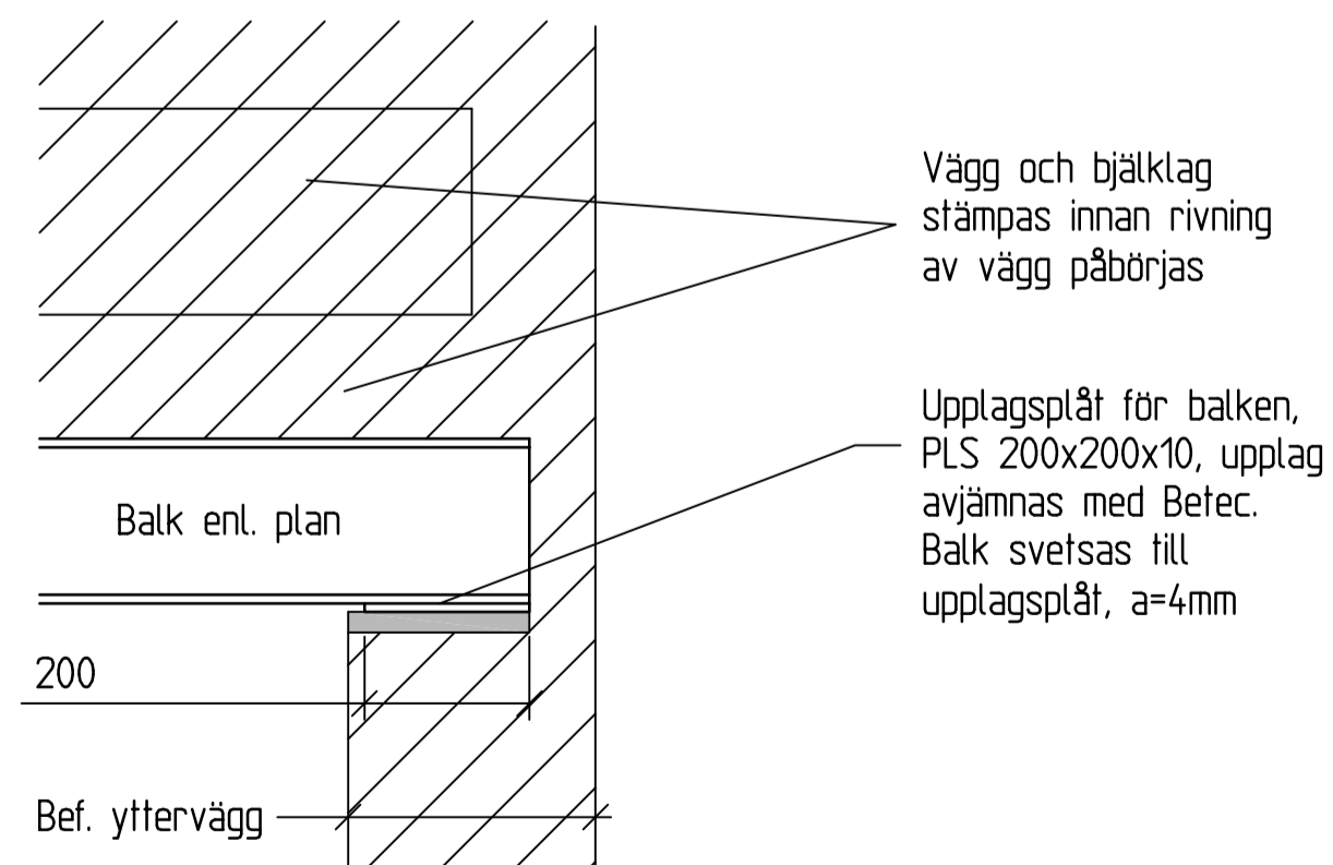
SEKTION C -1:10-
