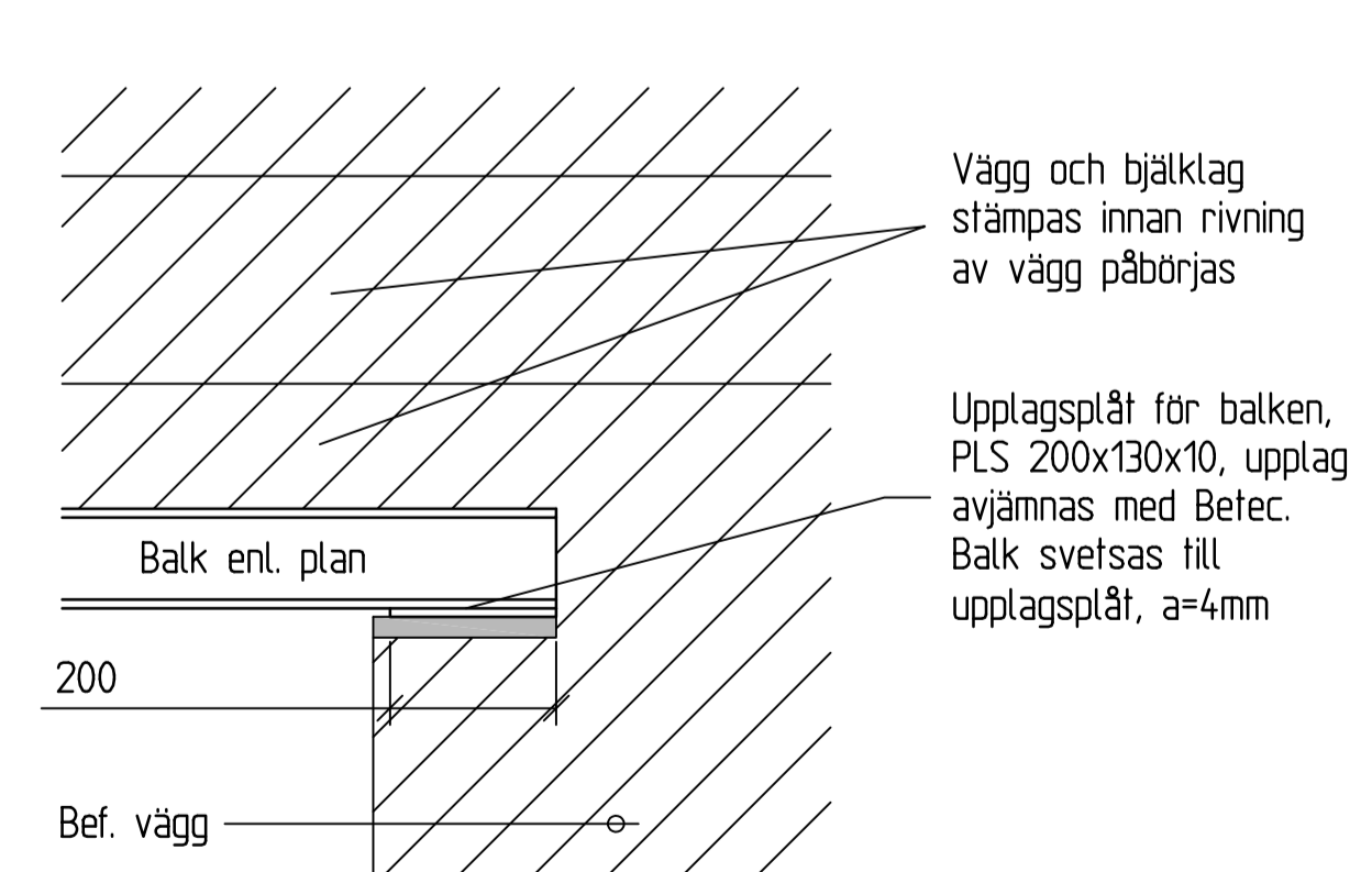
SEKTION E -1:10-
