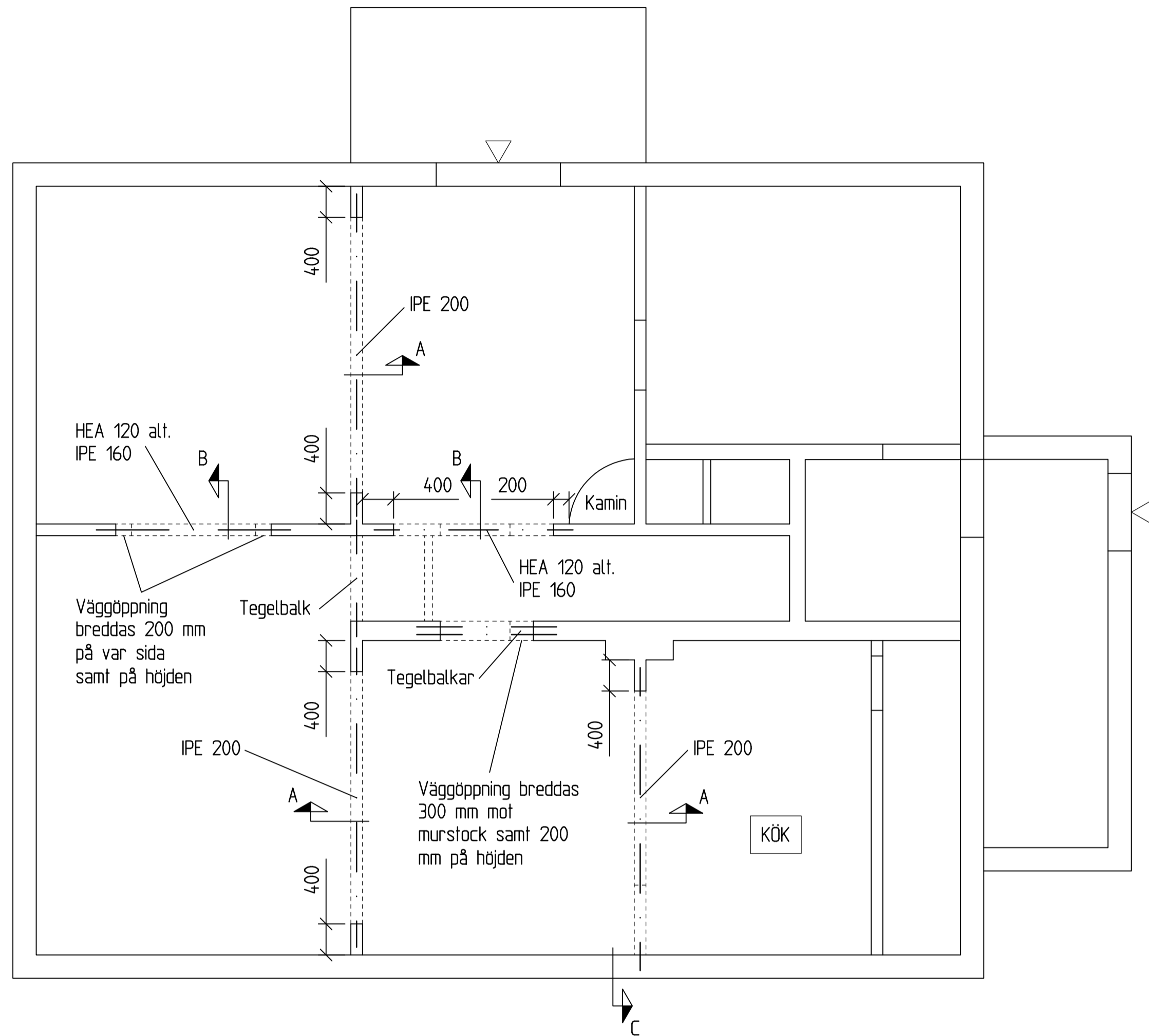
BJÄKLINGSPLAN -1:50-
