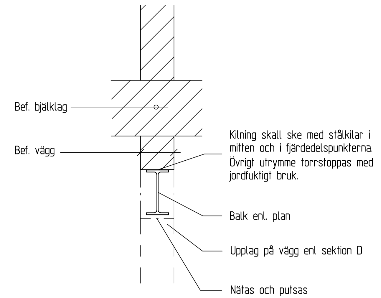
SEKTION A -1:10-
