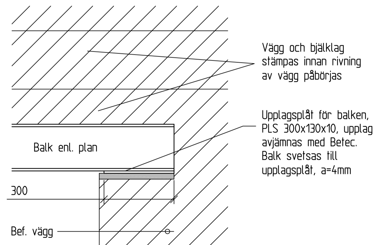
SEKTION D -1:10-
