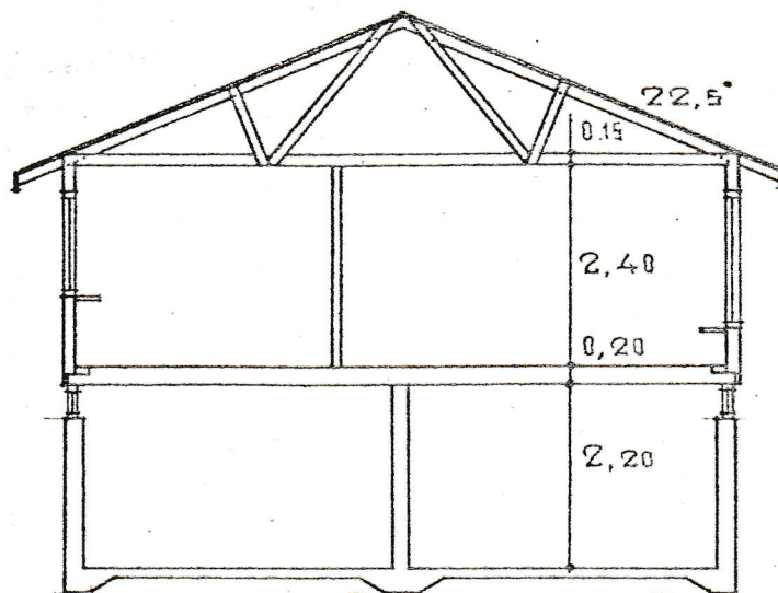
SEKTION KÄLLARE
