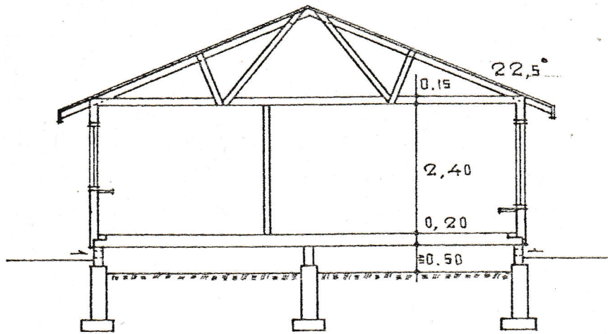
SEKTION KÄLLARLÖSA
