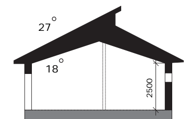
B-B 1:200
