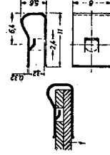
1.3 Fjädersförband
