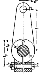
1.7 Klämförband
