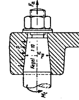
1.4 Koner
