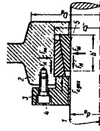
1.5 Spännelement
