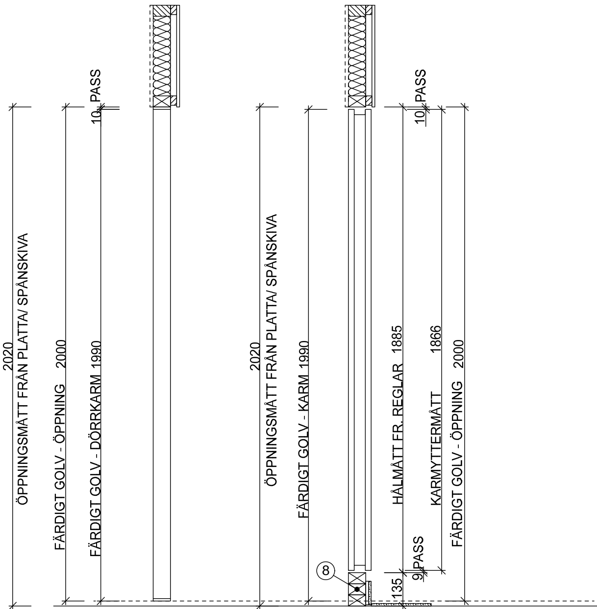
SNITT DÖRR (7x20) **/ KARMMÅTT : 690 x 1990
