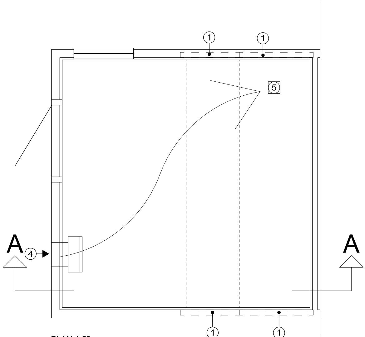
PLAN 1:50
