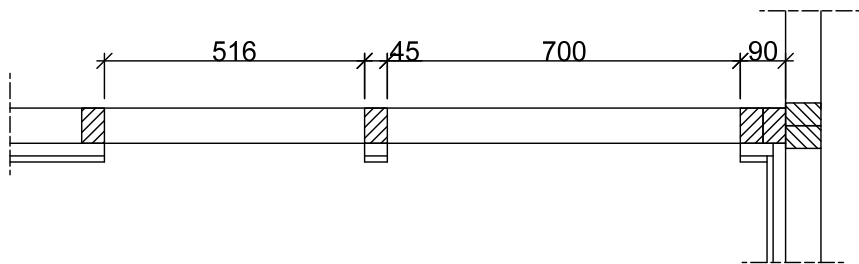
SNITT A-A
