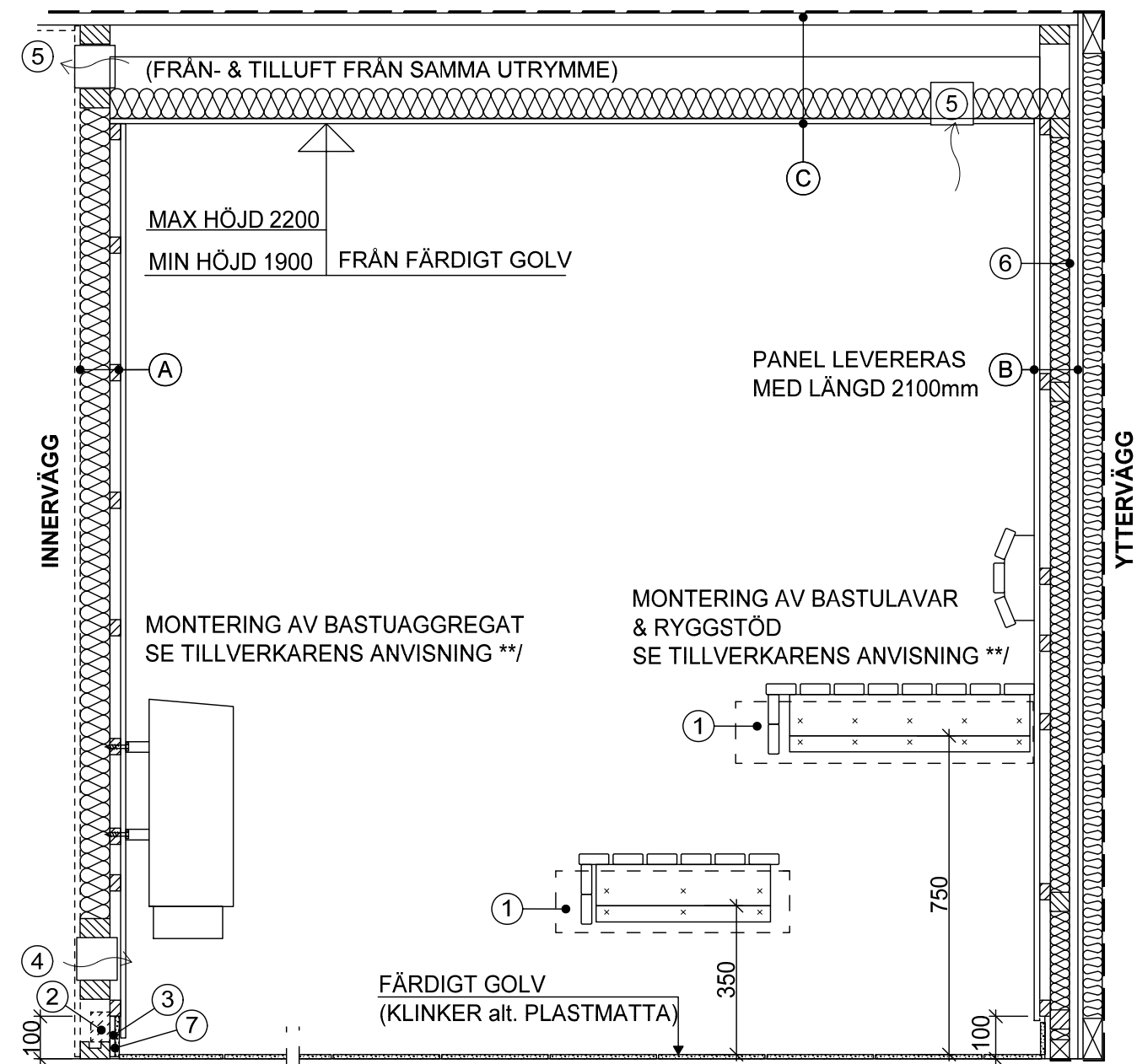
SNITT A-A
