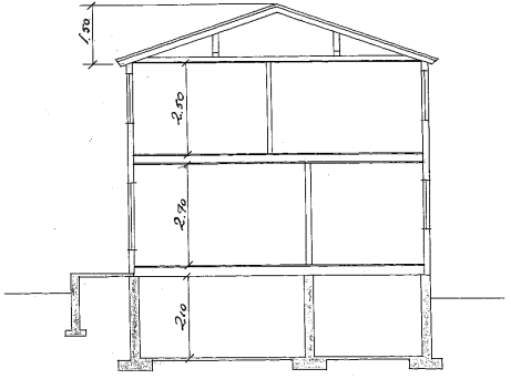
SEKTION
