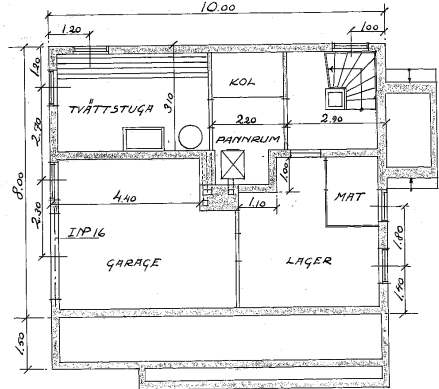
KÄLLARPLAN
