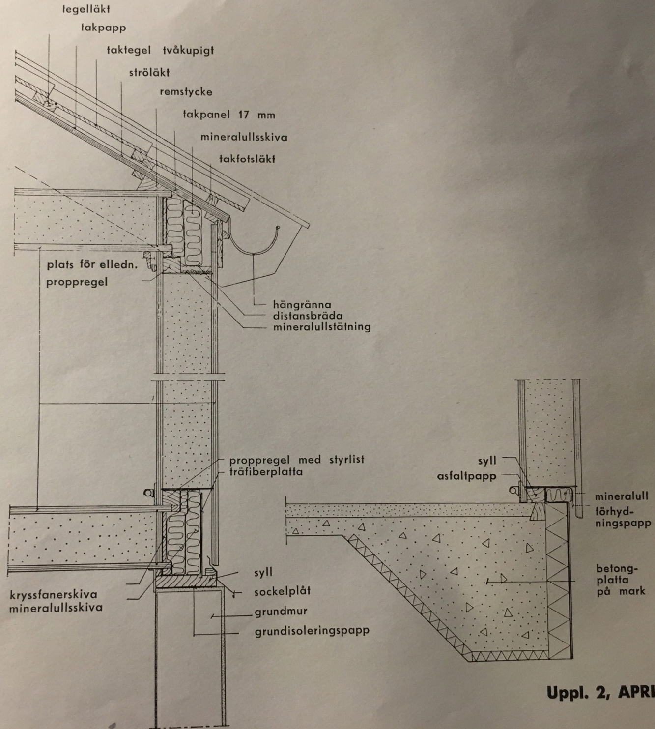
Figur 8. Vertikalsektion genom yttervägg och bjälklag
