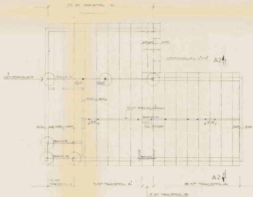
TAKSTOLSPLAN 1:100
