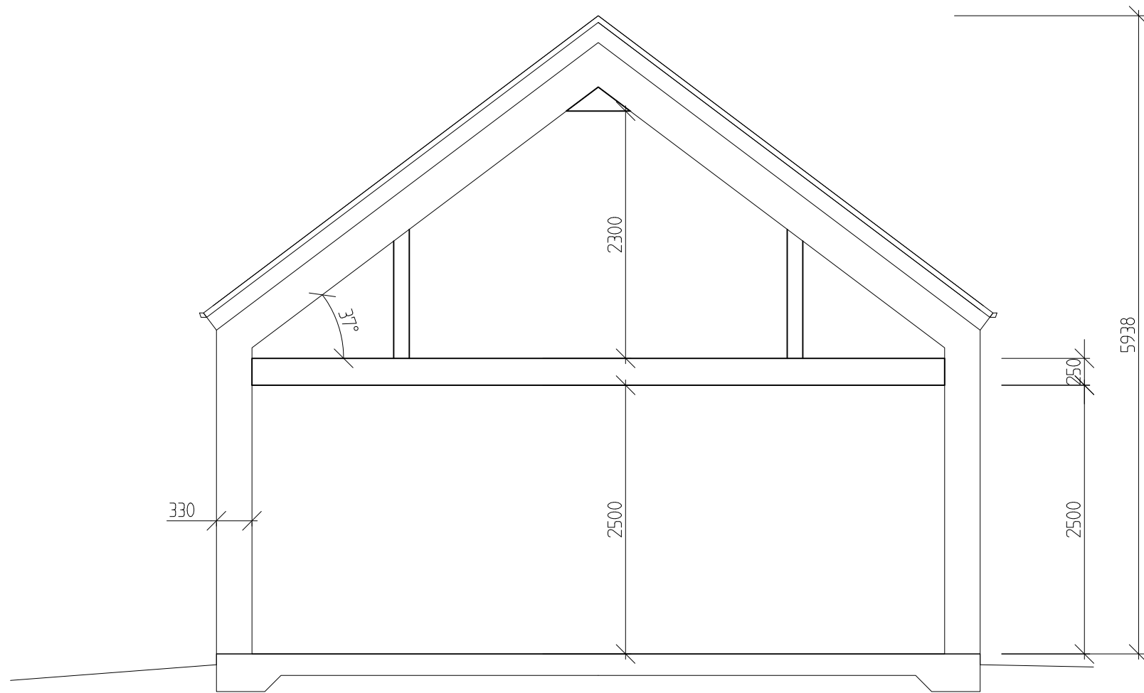
SEKTION A-A
