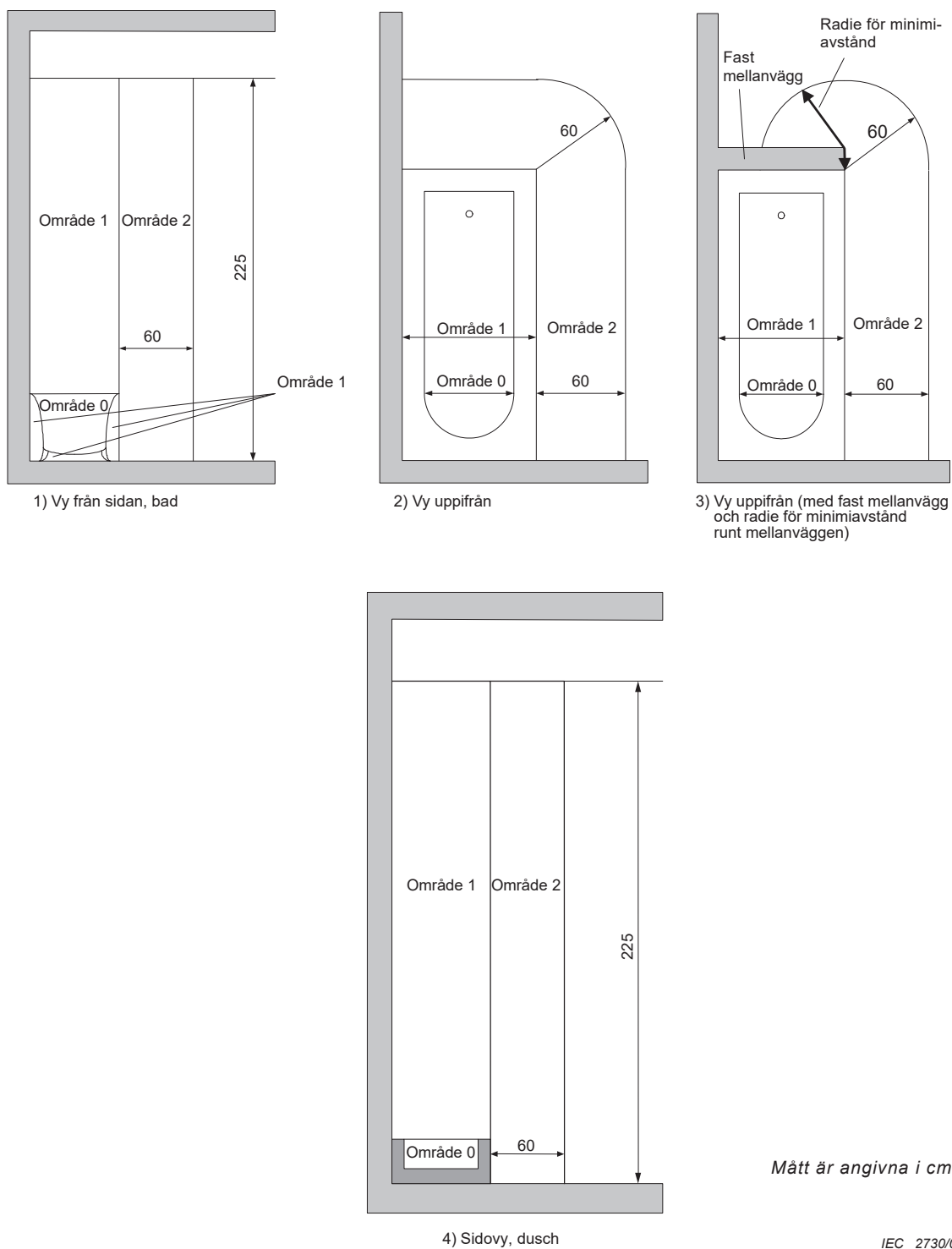
Figur 701.1 – Områdesindelning i badrum och duschrum
