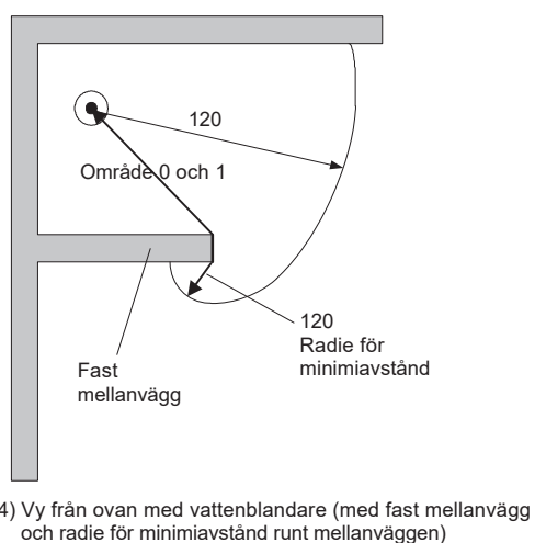
Figur 701.2 – Utbredning av områdena 0 och 1 i duschrum utan duschkar
