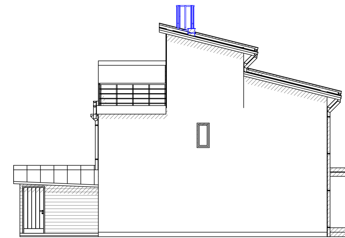
FASAD 2
