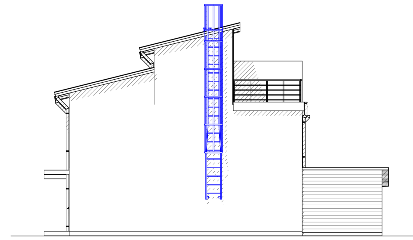
FASAD 4
