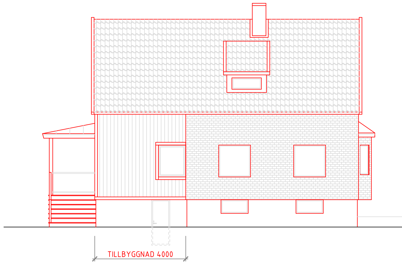
FASAD MOT VÄSTER
