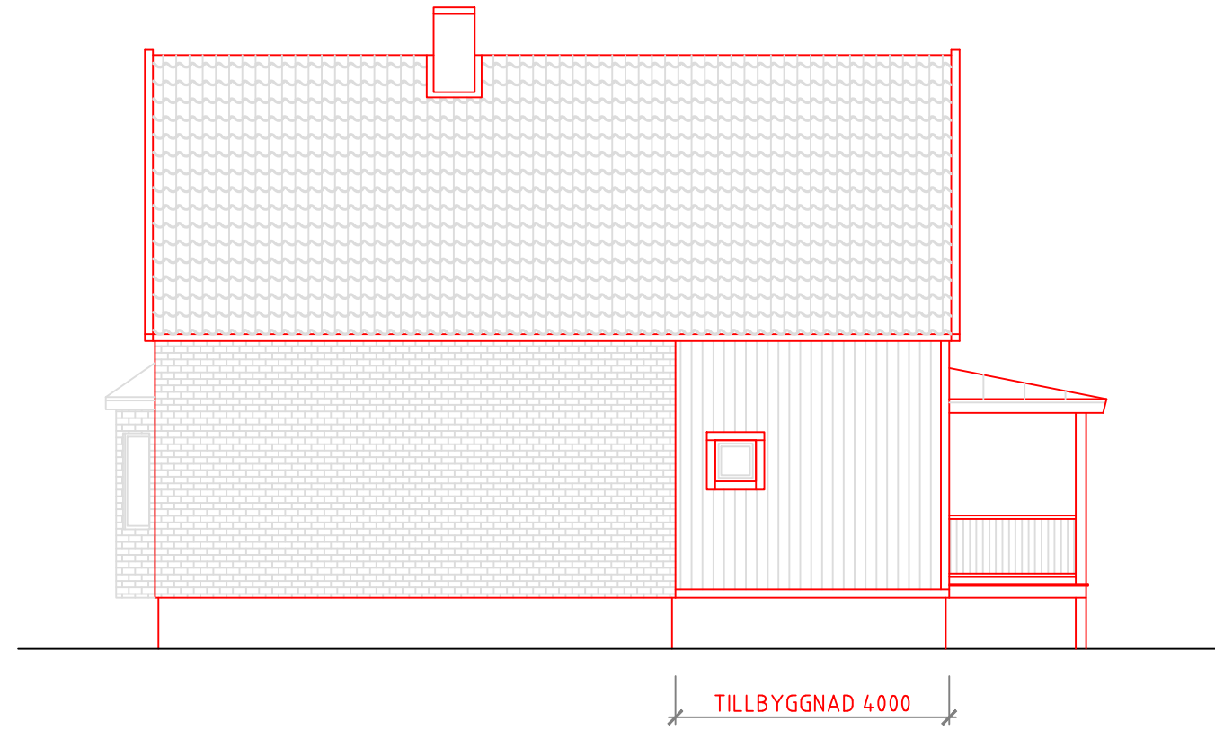
FASAD MOT ÖSTER
