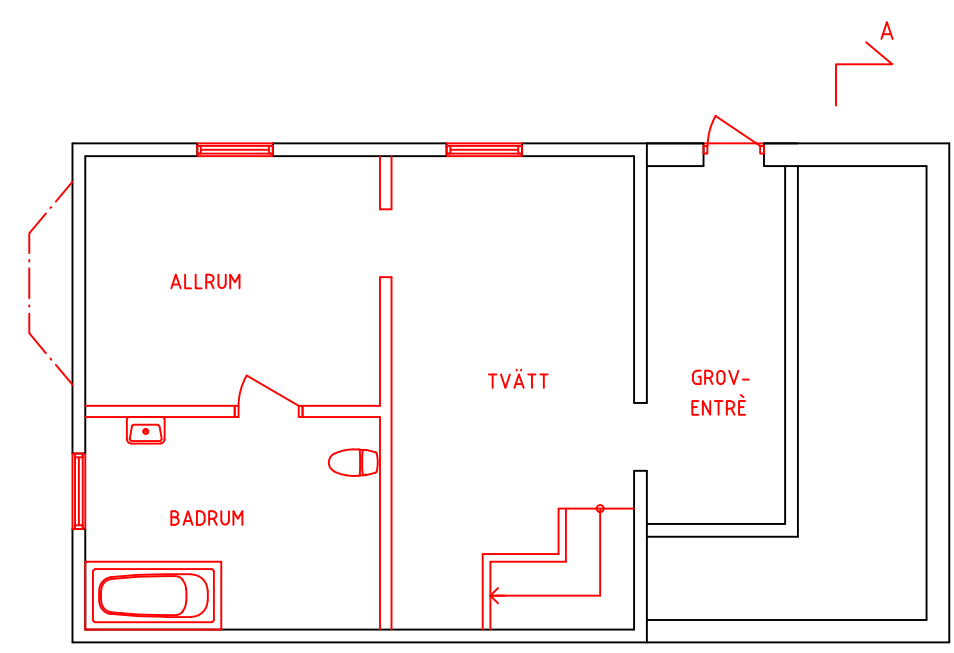
KÄLLARPLAN BOA: 54,9m 2 BYA: 76,5m 2
