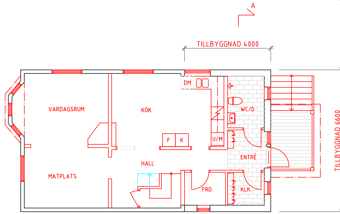
ENTRÉPLAN BOA: 69,7m 2 BYA: 77,7m 2
