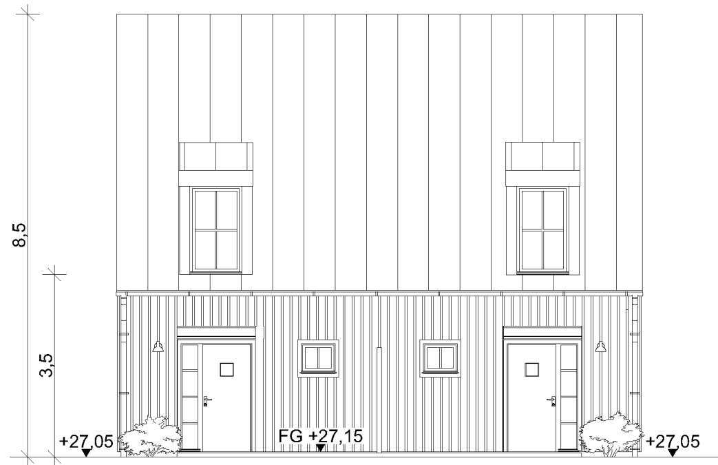
HUS 3 - FASAD MED ENTRÉER I SYDOST
