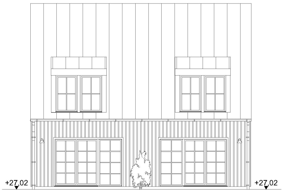
HUS 3 - FASAD MED UTEPLATSER I NORDVÄST
