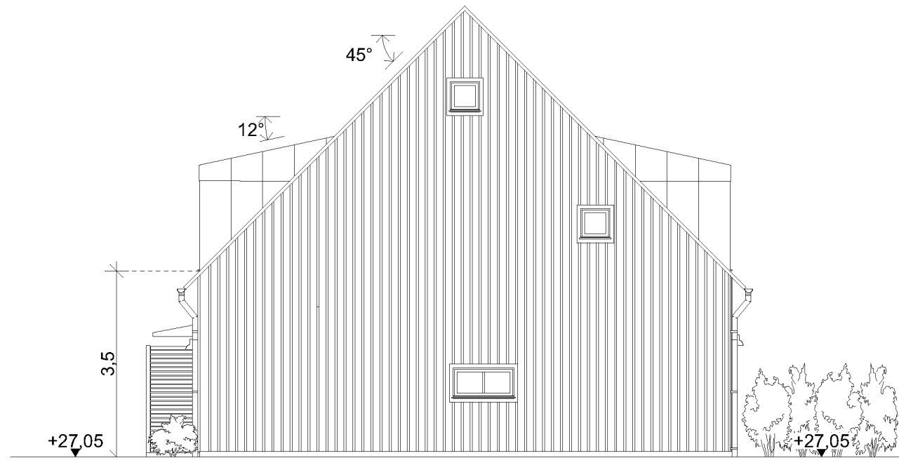
HUS 3 - FASAD MOT NORDOST
