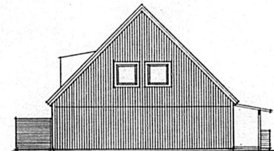
GAVELFASAD FÖNSTER I HUS 1006, 1009, 1120, 1122
